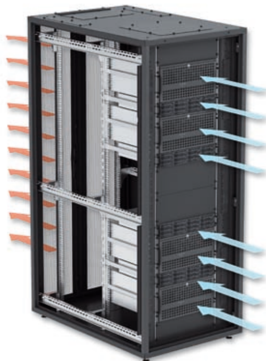
Шкаф с заглушками 19"
