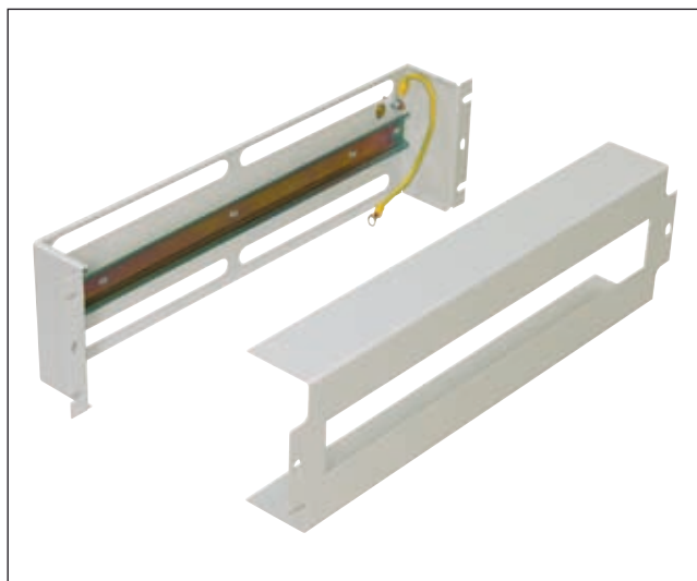
Панель 19" с DIN-рейкой
