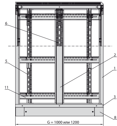
Разрез E-E
