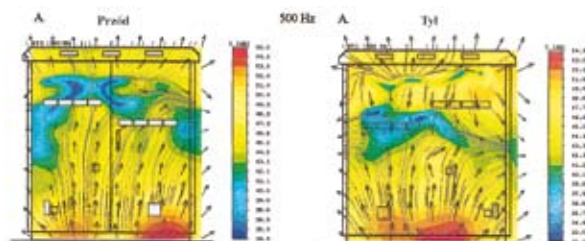
Rozkład pola wektorowego natężenia dźwięku dla tercji 500 Hz
