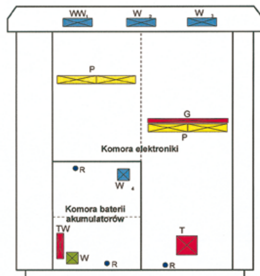
Rozmieszczenie wentylatorów w badanej szafie
