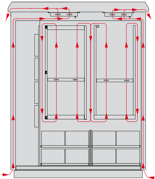
Schemat obiegu powietrza
